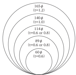
タフステン断面寸法図
