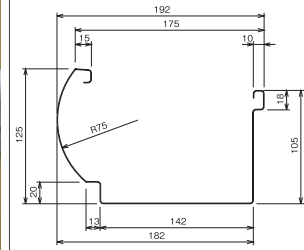
タフゾウ断面寸法
