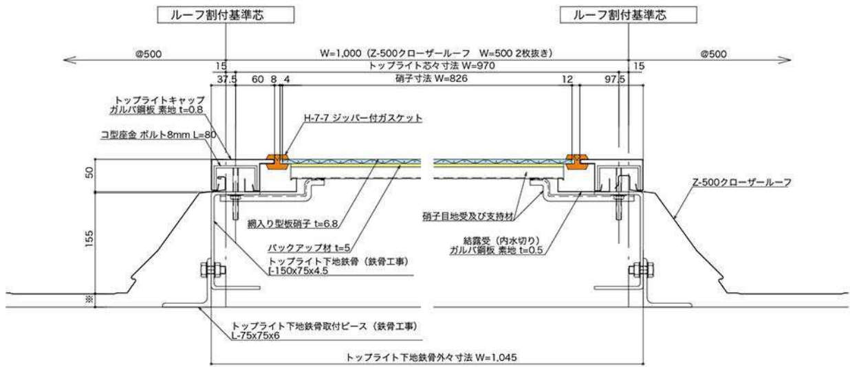
SH-1型 Z-500クローザールーフ用トツプライト 下地不要タイプ
