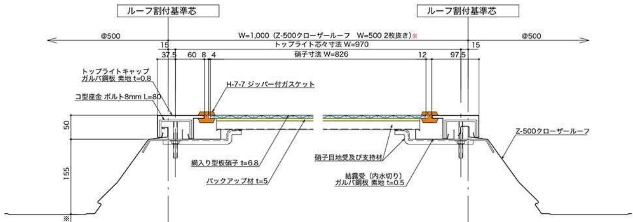
SH-1型 Z-500クローザールーフ用トツプライト 下地不要タイプ
